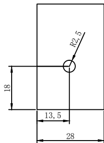
金属外壳一
