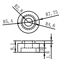
陶瓷垫片二
