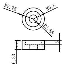
陶瓷垫片一
