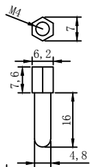
金属螺杆
