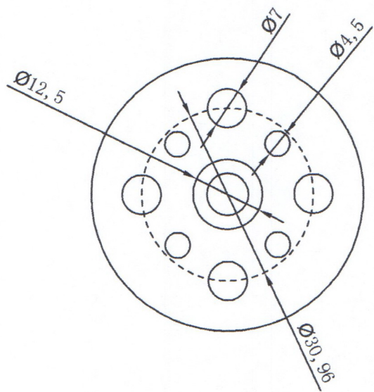
仰视图
